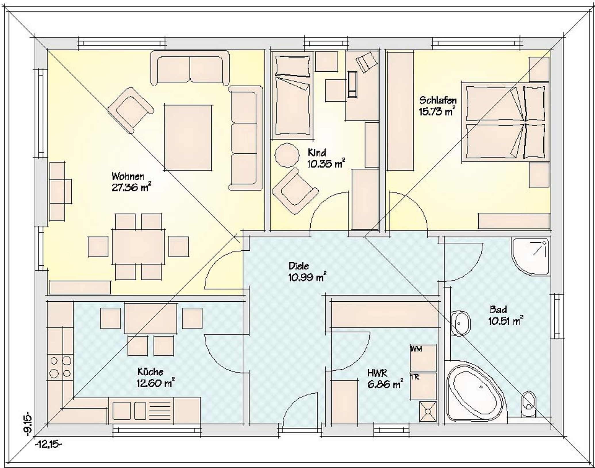
Erdgeschoss
