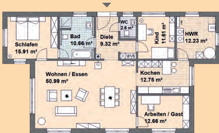
Grundrissvariante 2
