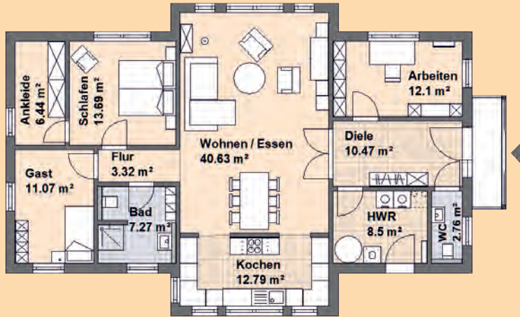
Grundrissvariante 1
