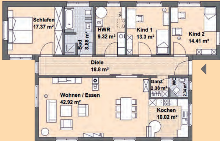
Grundrissvariante 1
